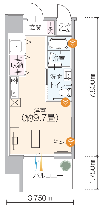
居室間取図(一例)
