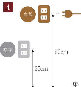
4 コンセント・スイッチを 負担の少ない位置に設計
